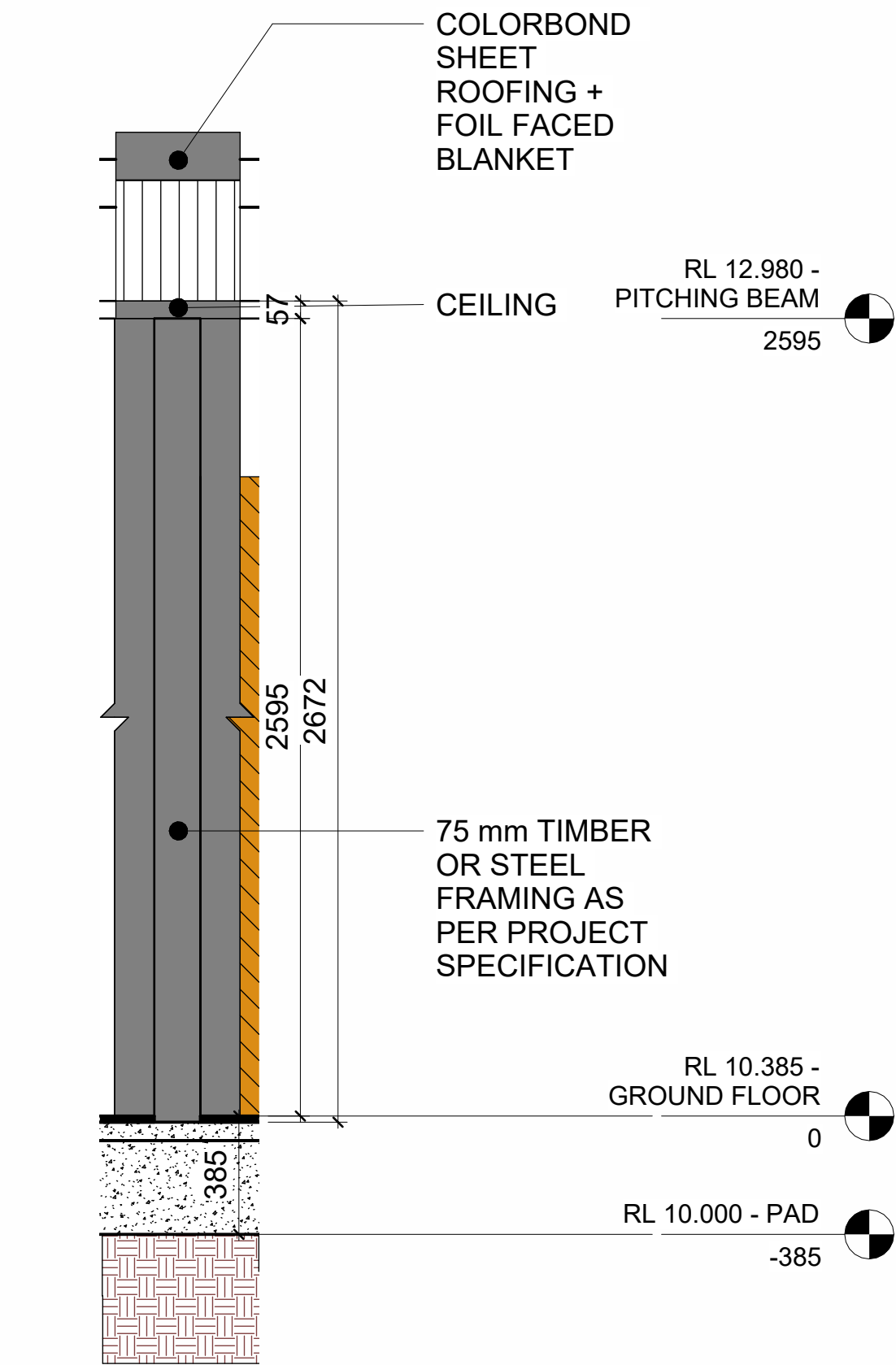
2 WALL SECTION 2 1 : 20
