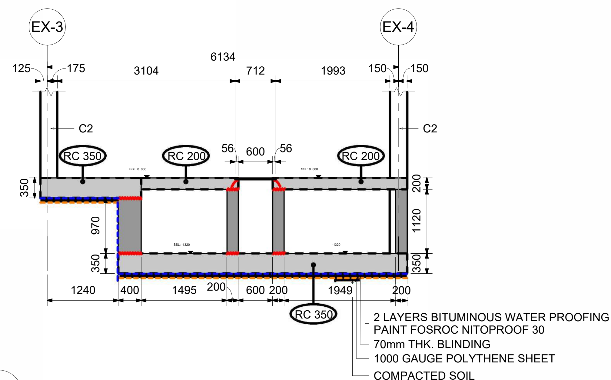
E Section E 1 : 40
