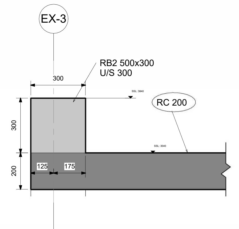
③ Section 7 1 : 10
