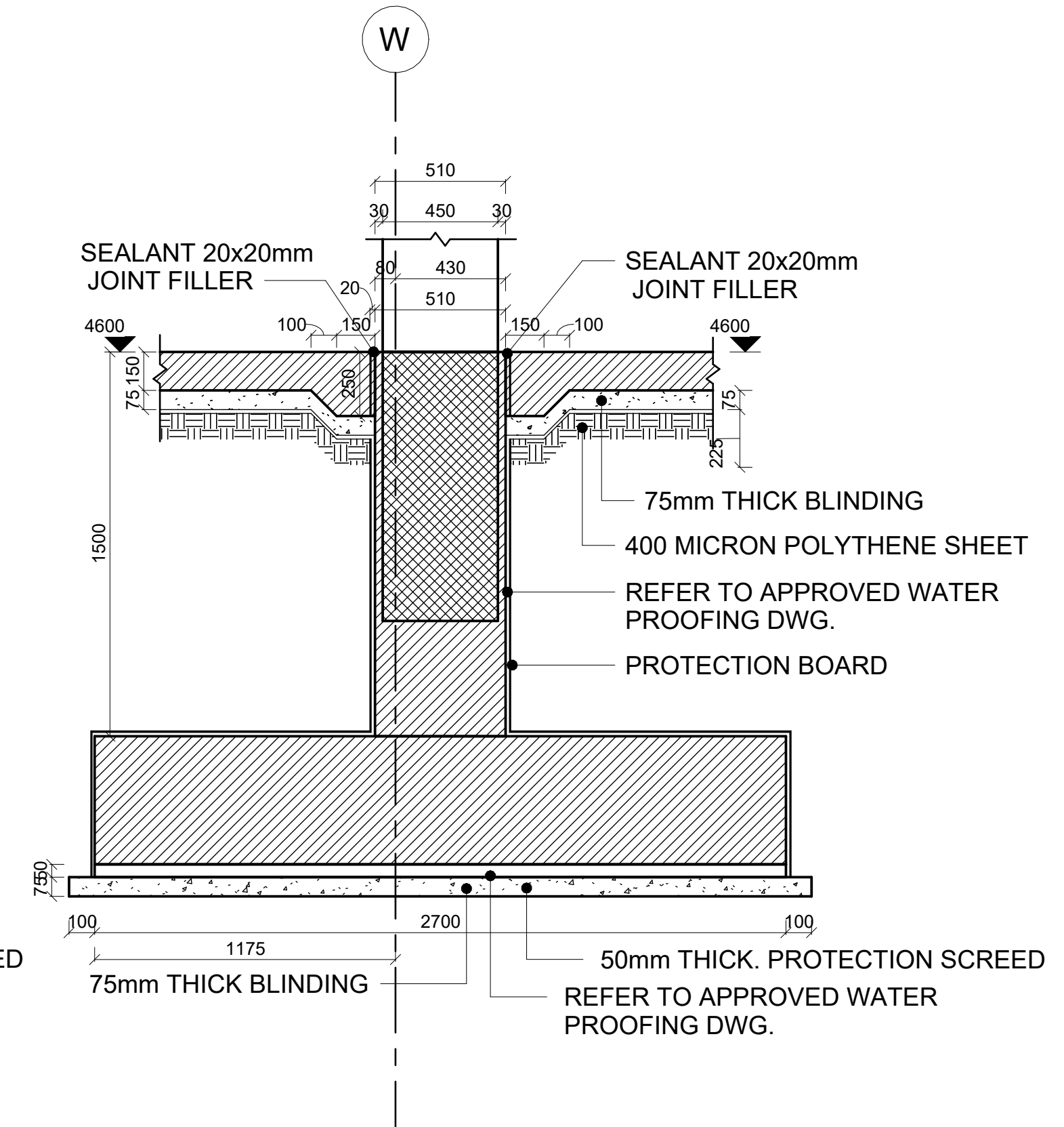
4 SECTION-04 (F2) DETAIL 1 : 20
