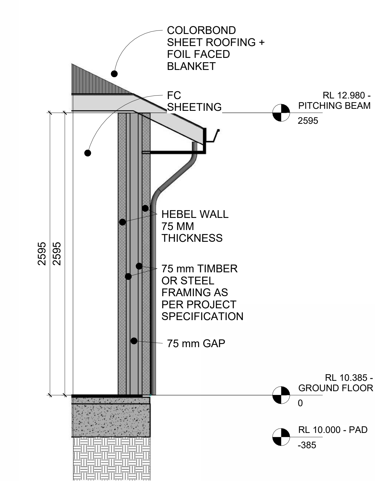
3 WALL SECTION 3 1 : 20
