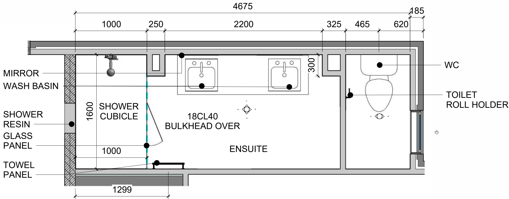
ENSUITE/WC PLAN 1 : 25
