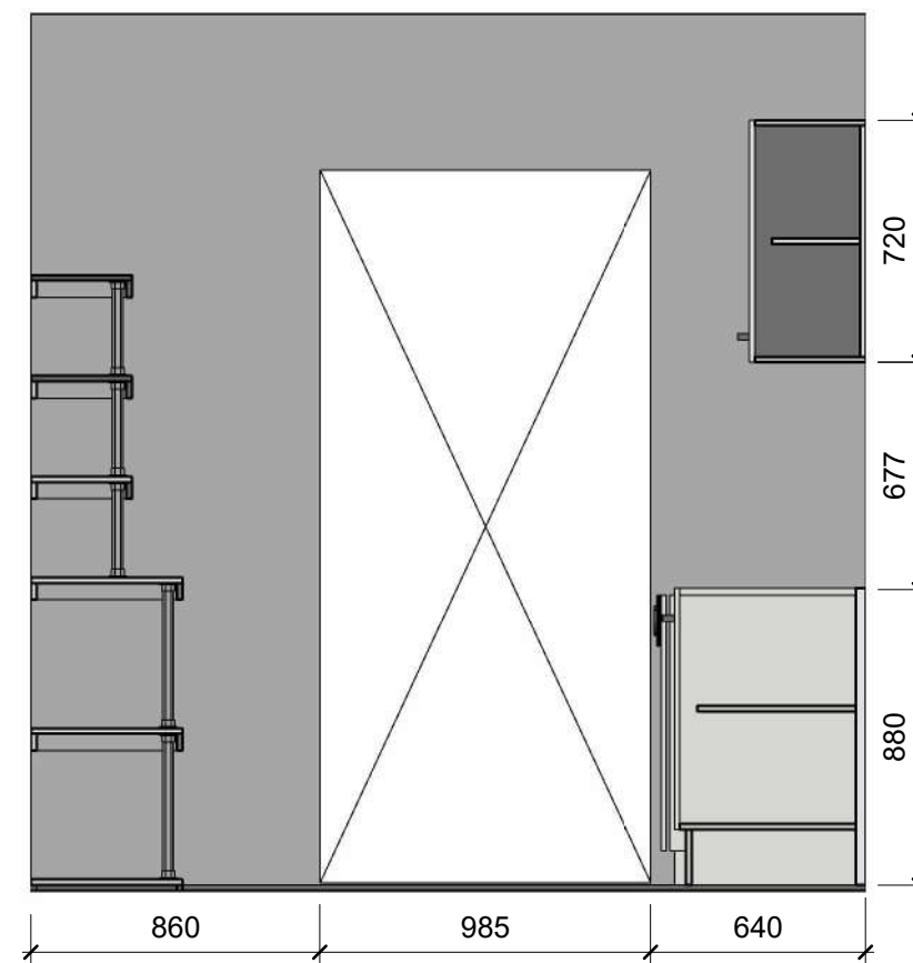
6 ELEVATION E 1 : 25
