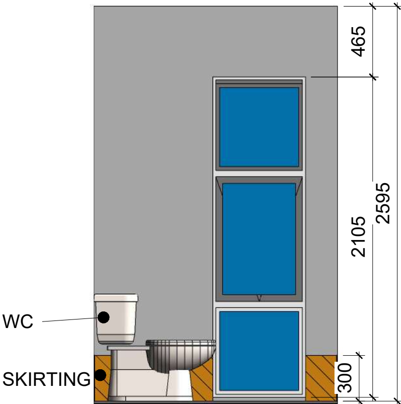
ELEVATION F1 1 : 25
