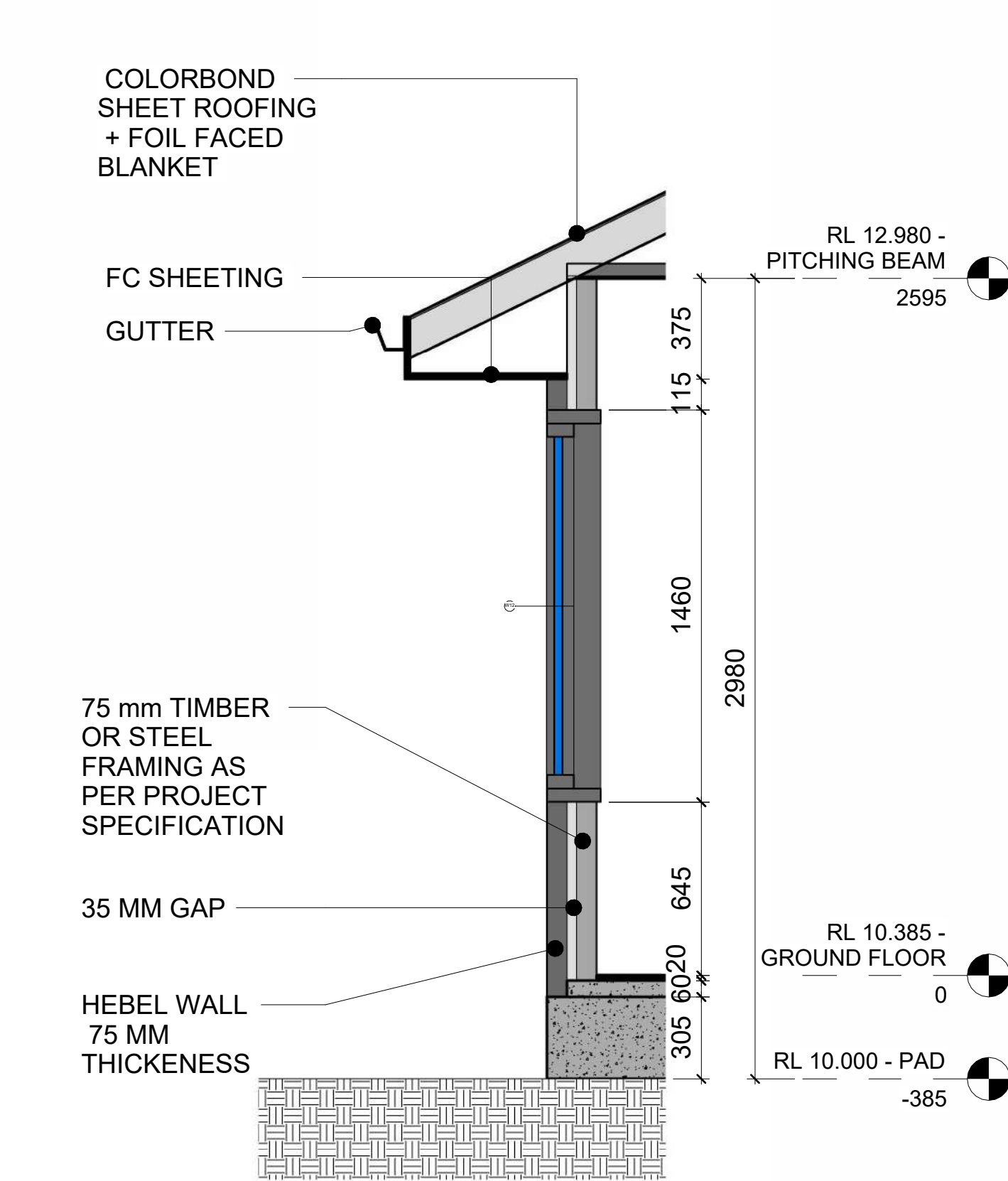
1 WALL SECTION 1 1 : 20
