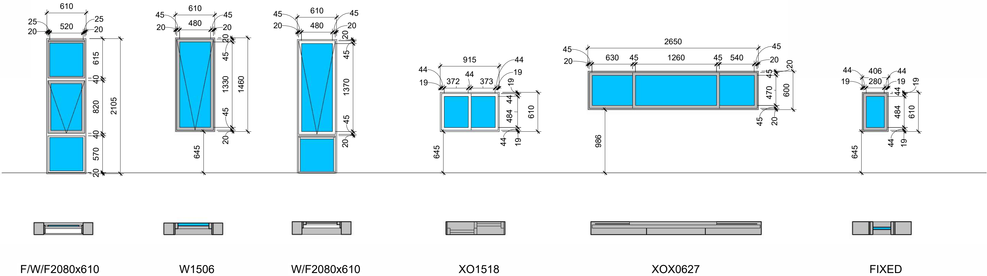
WINDOW LEGEND 1 : 35
