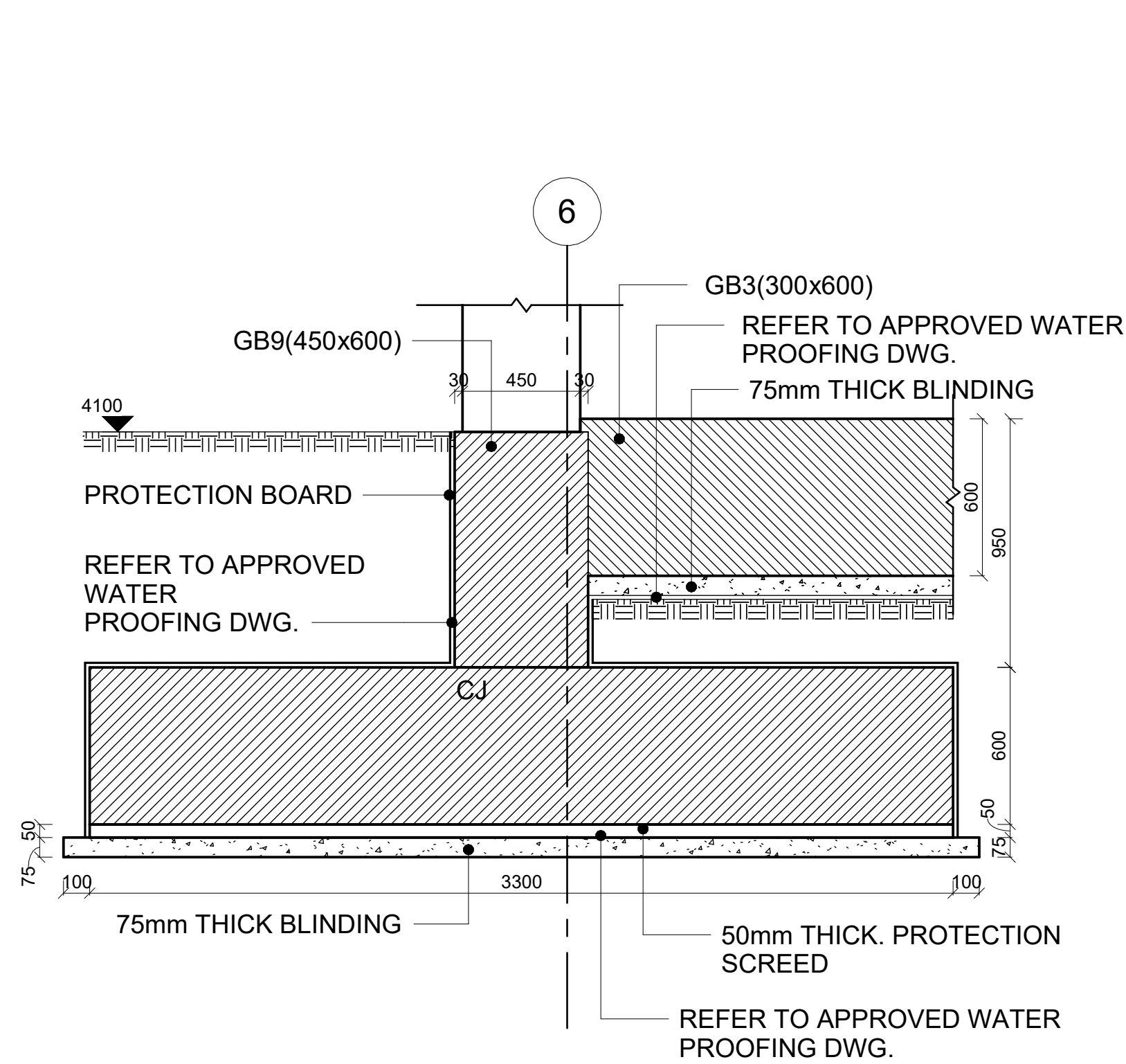
1 SECTION-01 (F1) DETAIL 1 : 20
