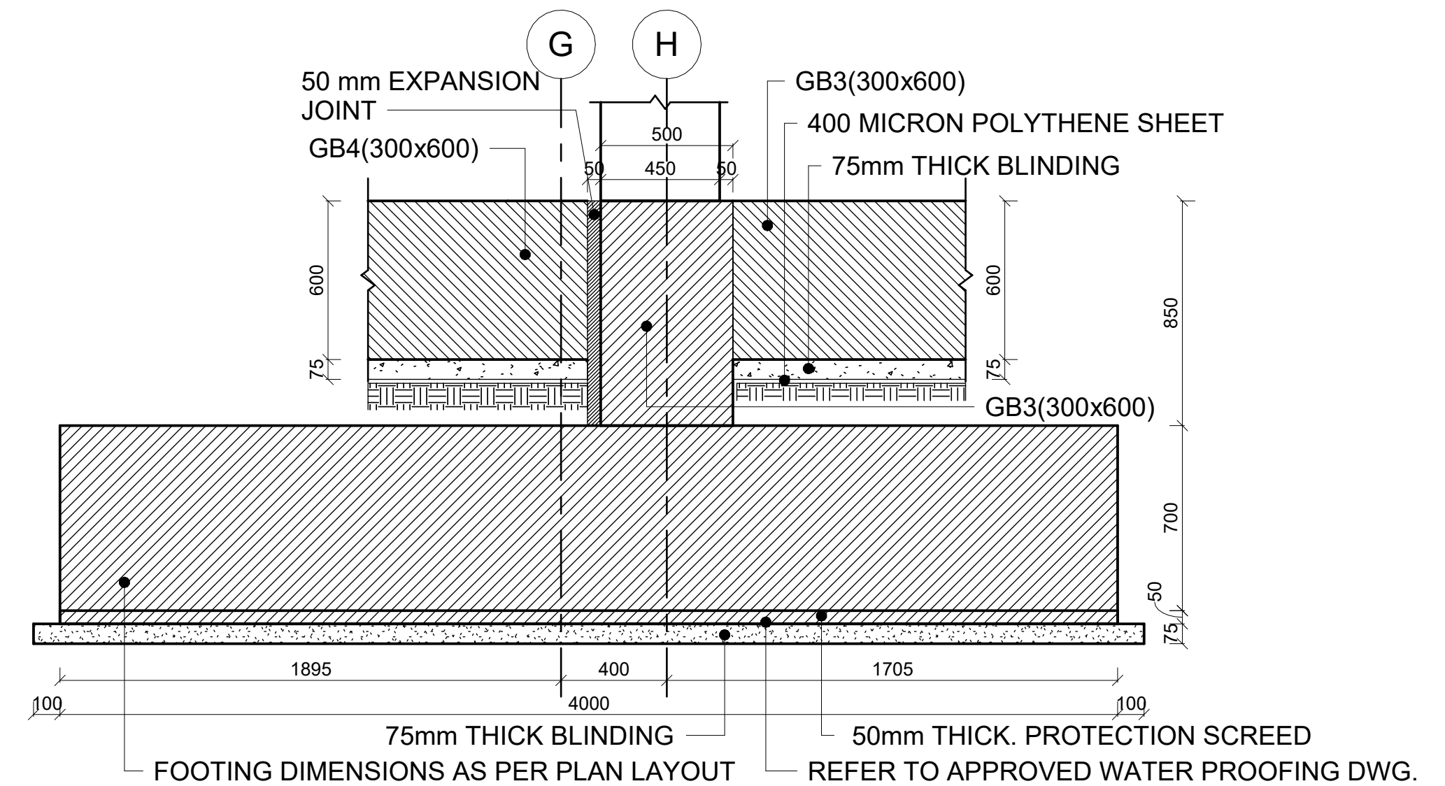
13 SECTION-13 (F10) DETAIL 1 : 20
