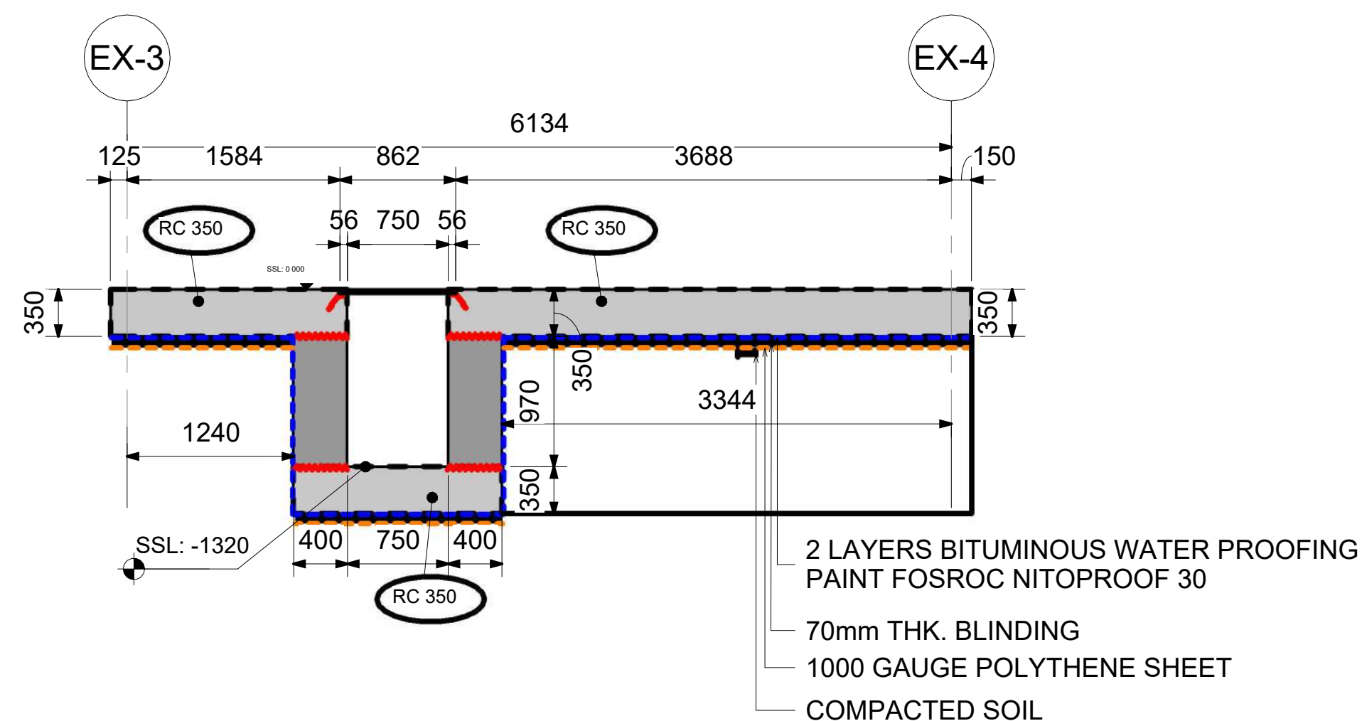
D Section D 1 : 40
