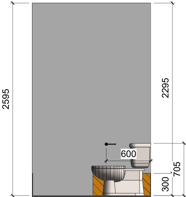
ELEVATION E1 1 : 25
