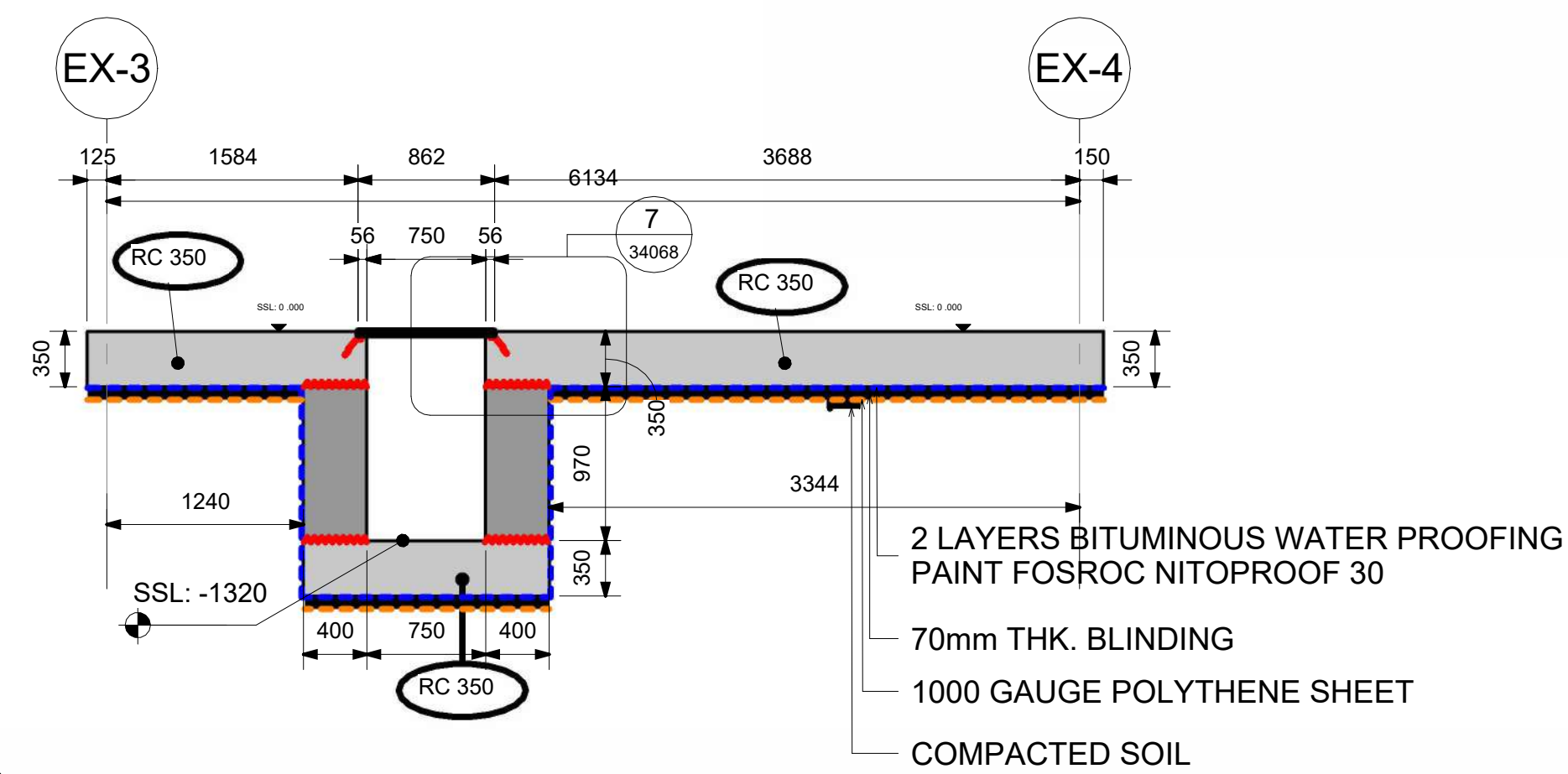
A Section A 1 : 40
