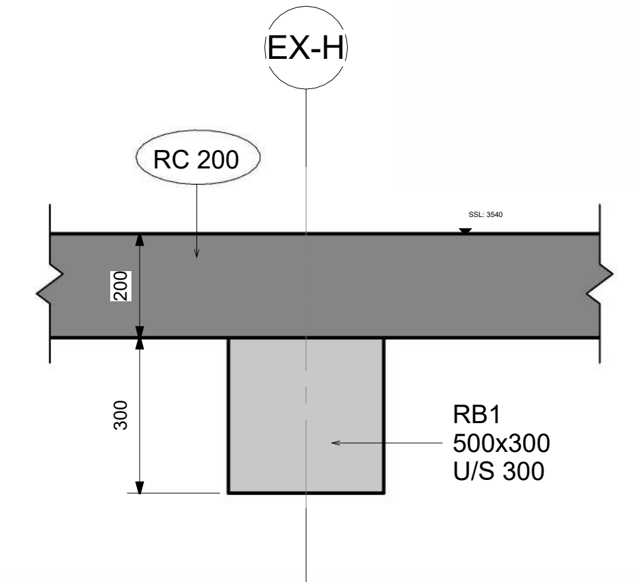
④ Section 8 1 : 10
