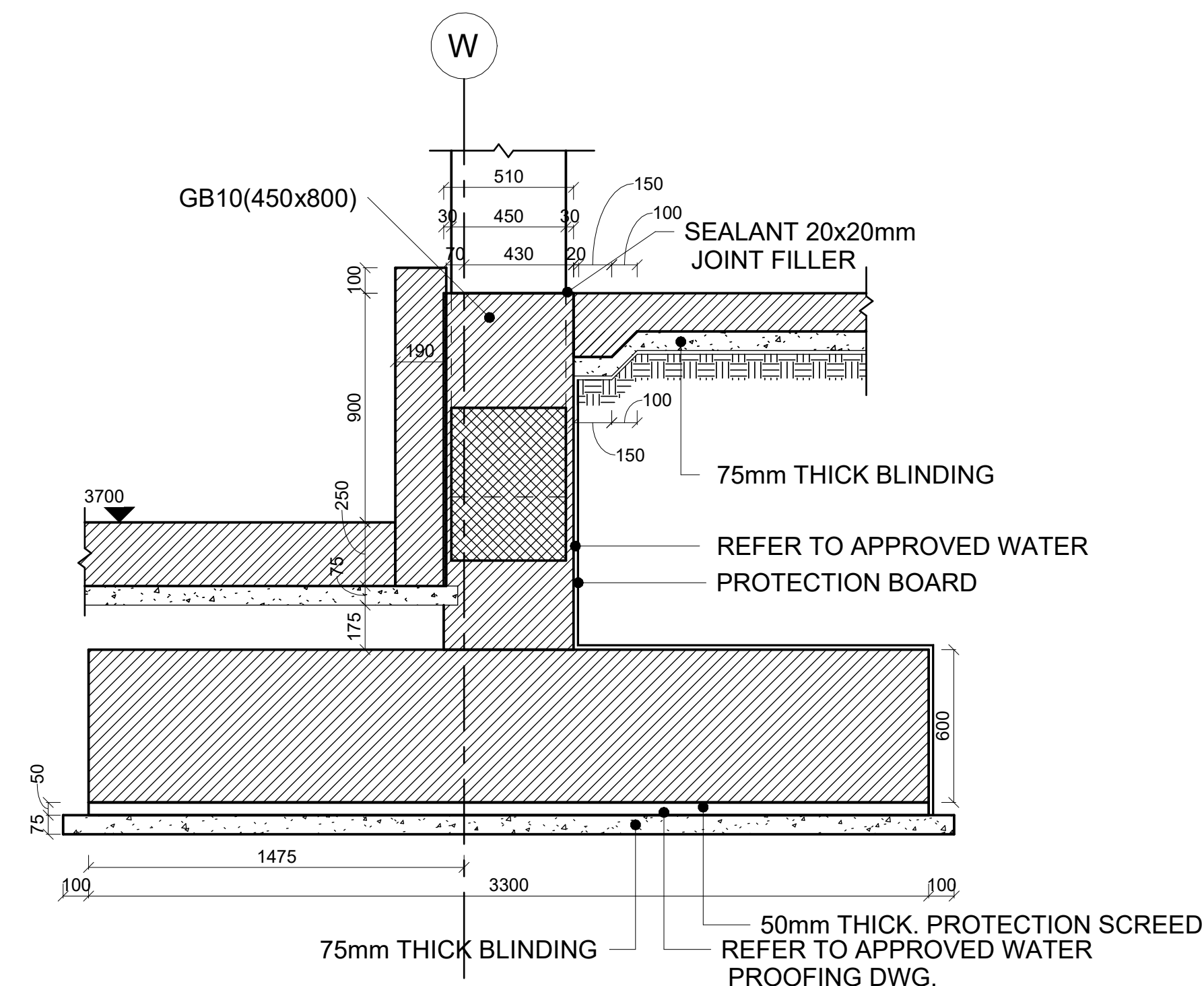
2 SECTION -02 (F1) DETAIL 1 : 20
