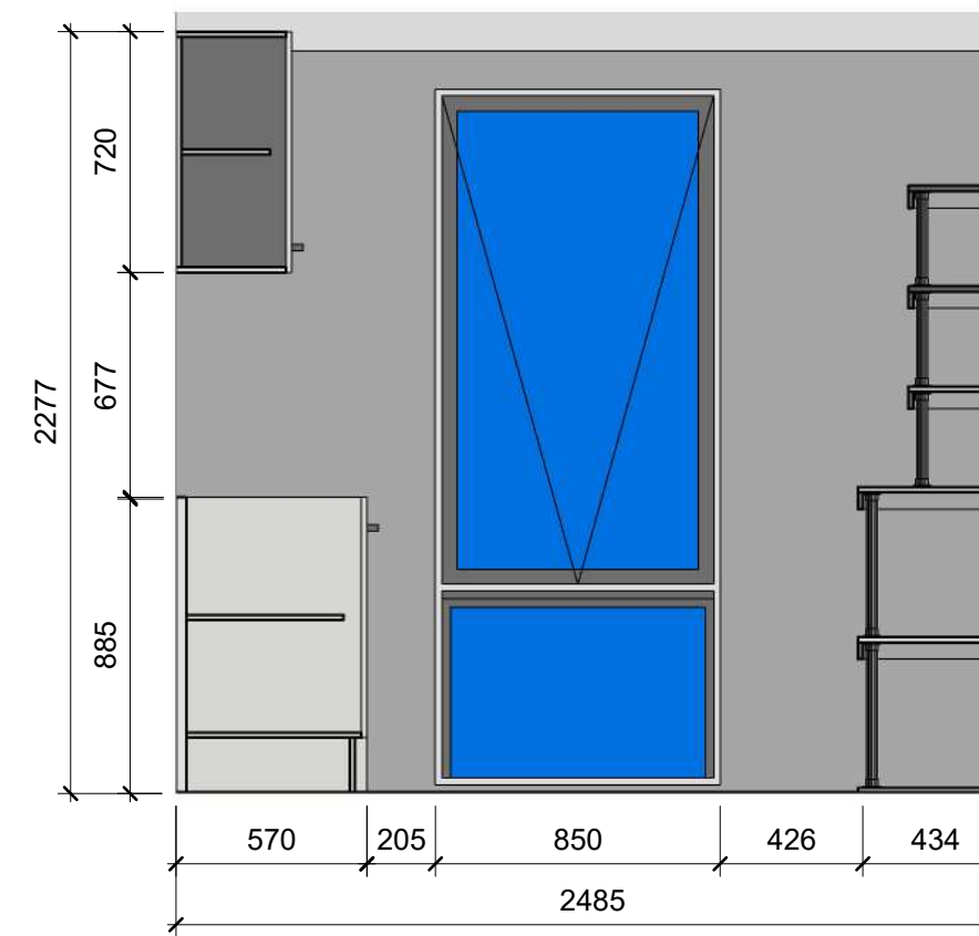
2 ELEVATION F 1 : 25
