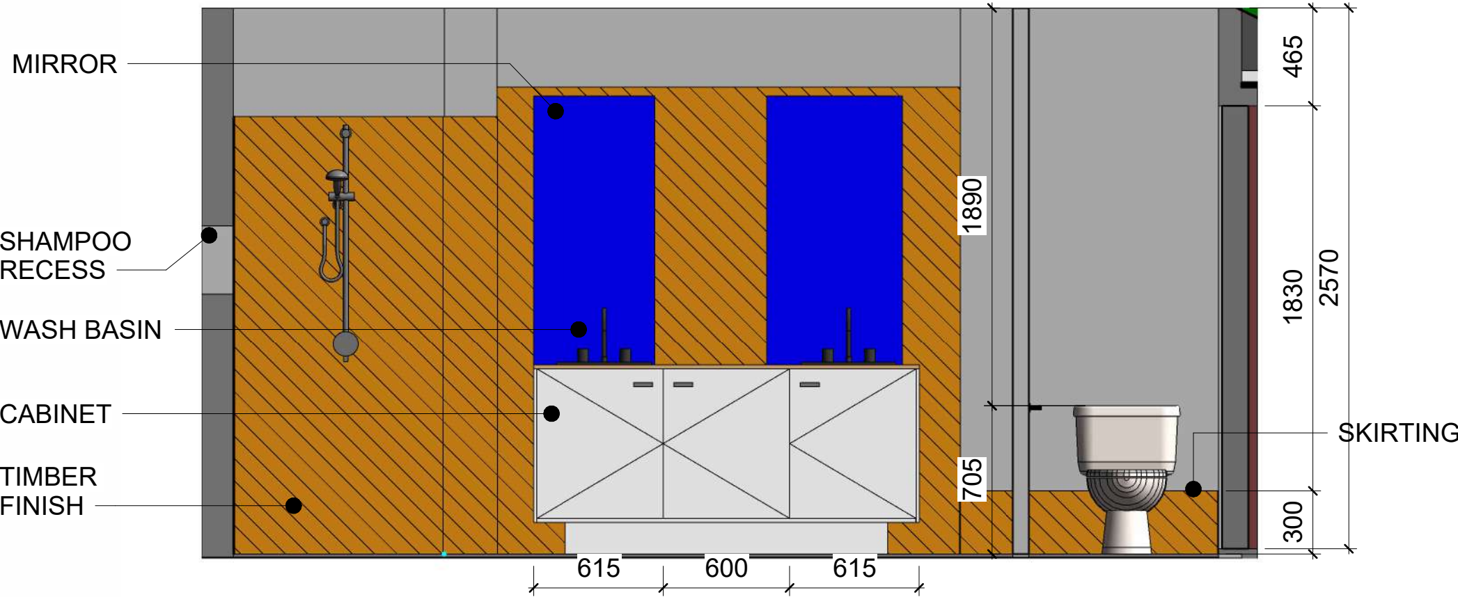
ELEVATION A1 1 : 25
