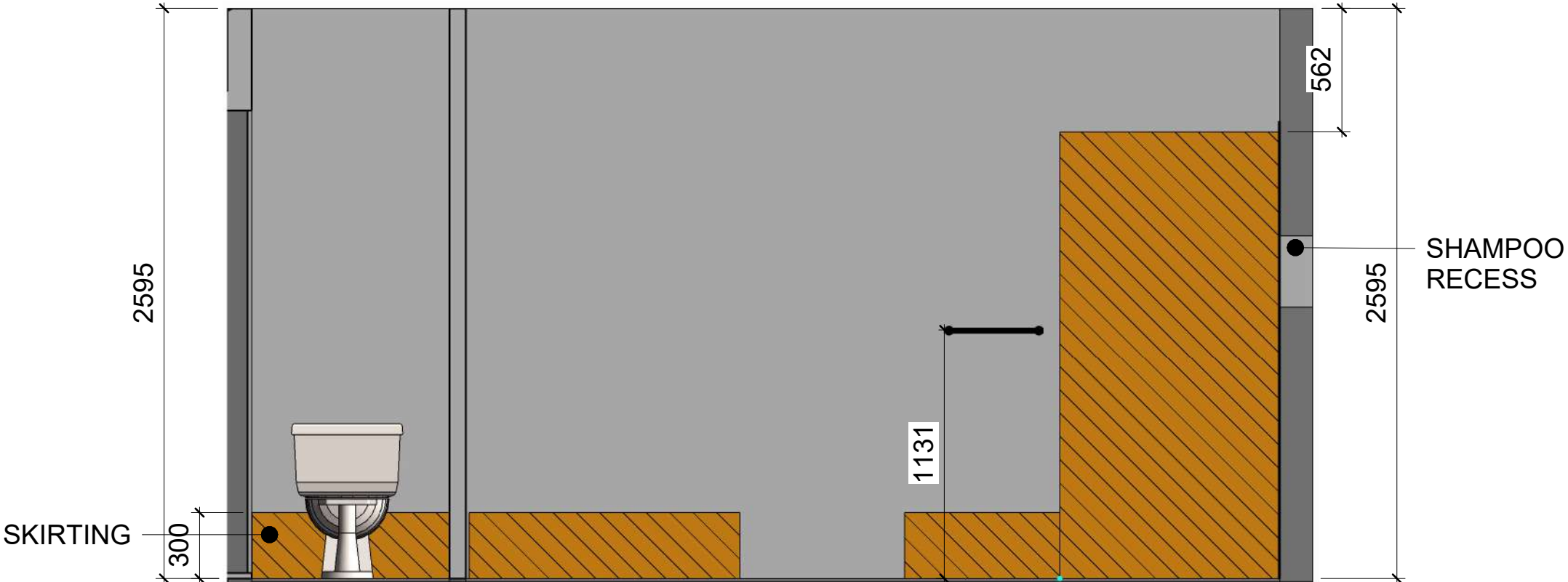
ELEVATION C1 1 : 25
