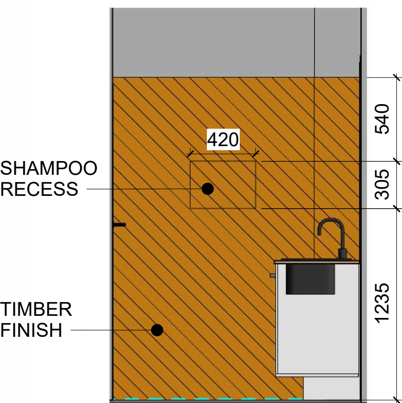
ELEVATION D1 1 : 25
